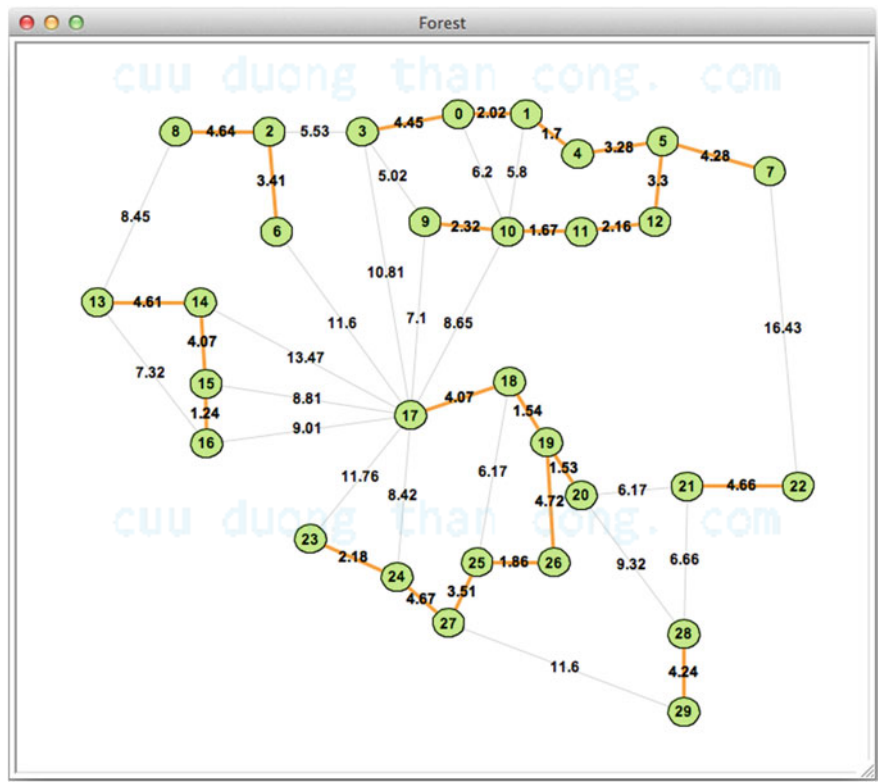
Fig. 7.6 Kruskal’s: Snapshot 1
